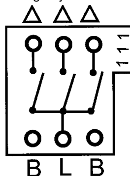
Koblingsskjema
