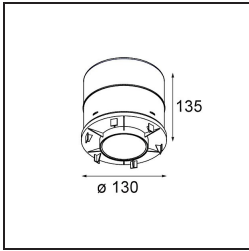
12339930 Conbox Ø130x135
