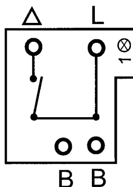
Koblingsskjema
